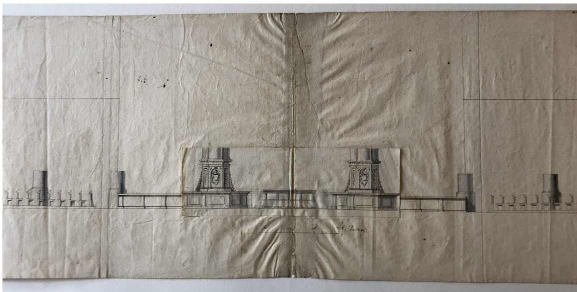
Ontwerptekening uit 1661 van Willem van der Helm. Dwarsdoorsnede transept gezien richting het westen. In het schip en noorder- en zuidertransept zijn vaste banken getekend. (collectie ELO)
